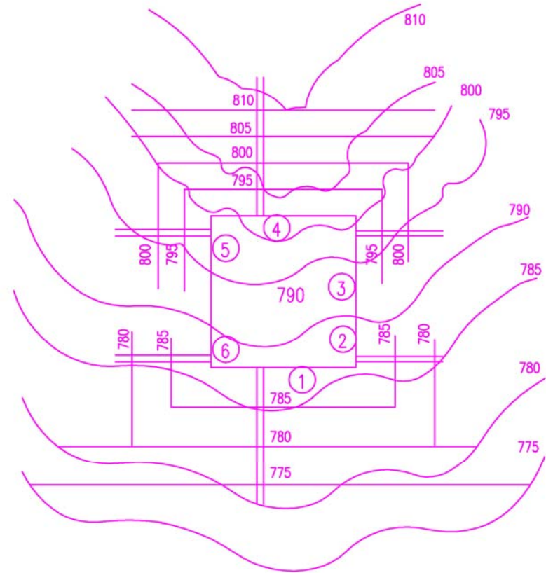
Identificación de taludes y horizontales a equidistancia
