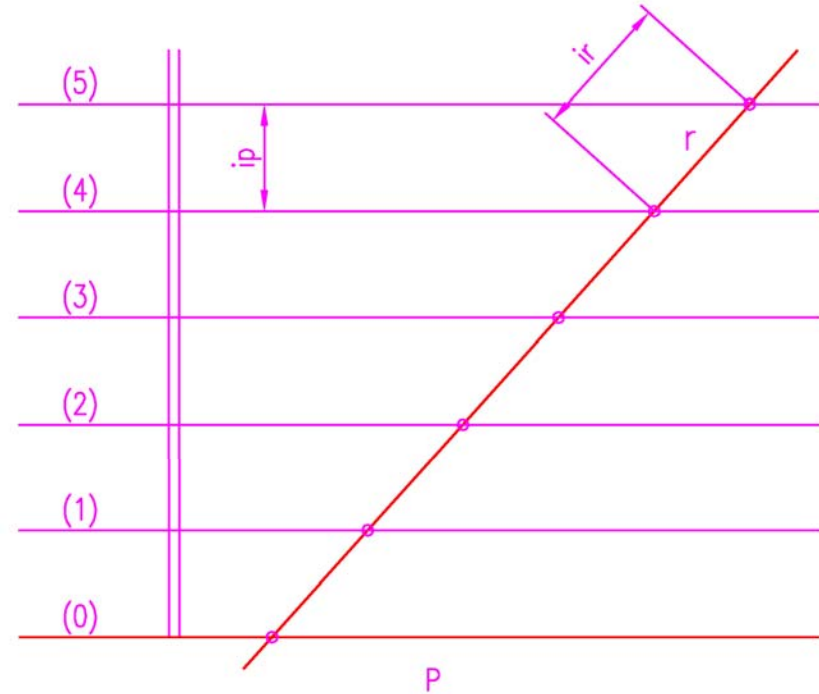
Intervalo de recta en plano
