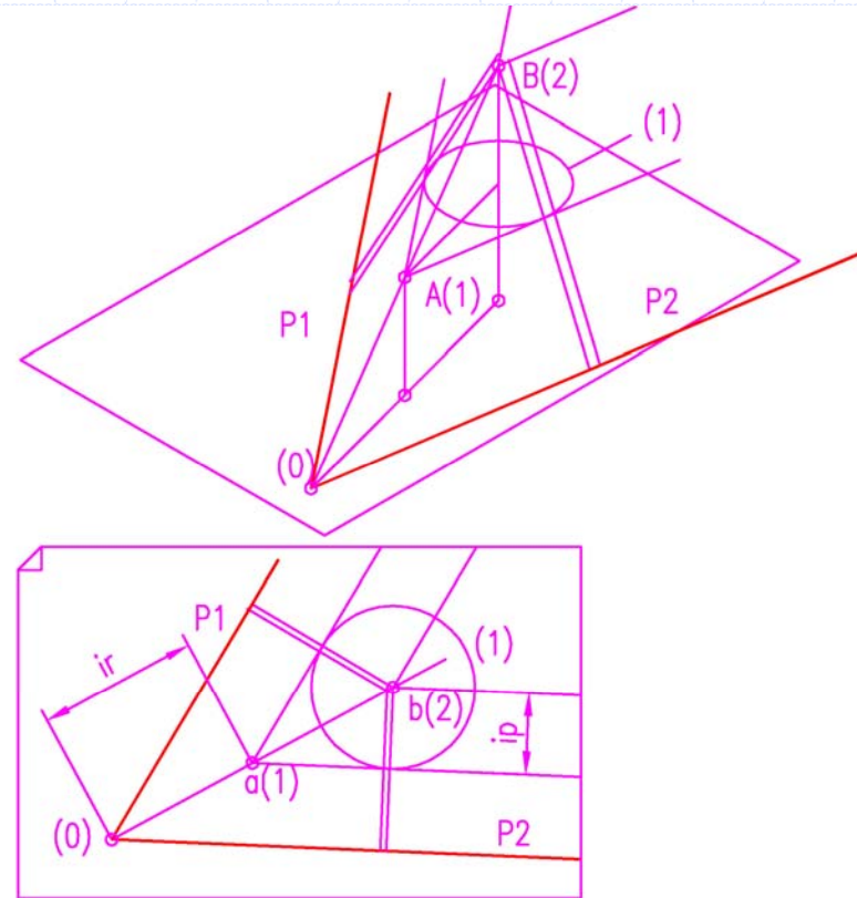
Trazar un plano de intervalo dado conteniendo a una recta
