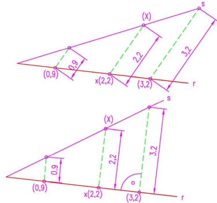
Cálculo de la cota de un punto
