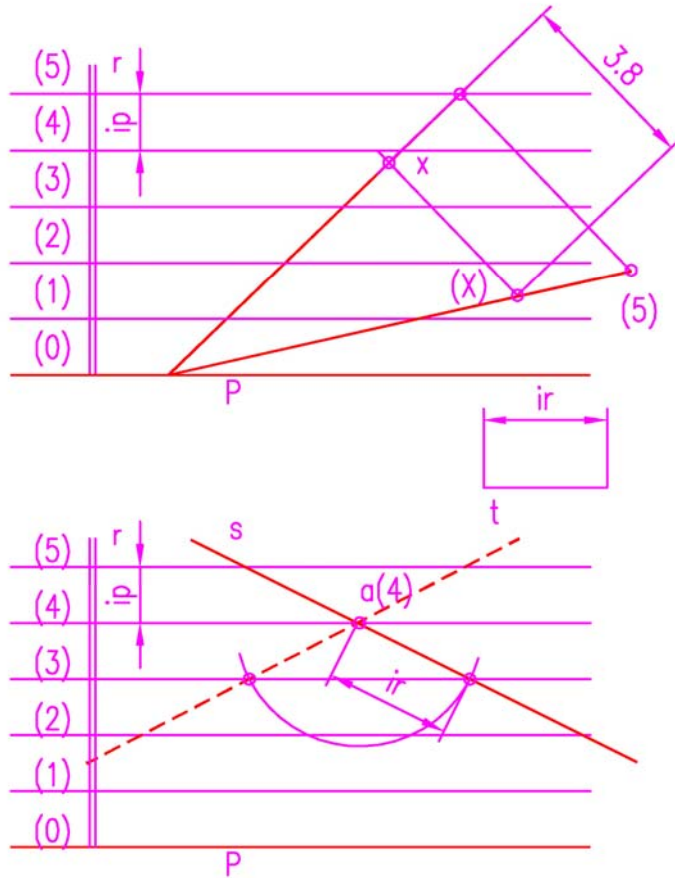
Cota de un punto en un plano. Trazar recta contenida en un plano
