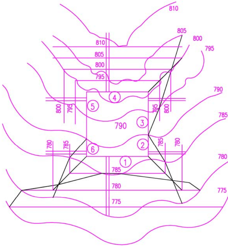
Trazado de intersecciones entre taludes y con el terreno
