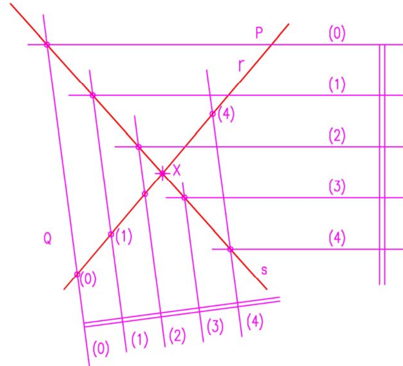
Intersección entre recta y plano
