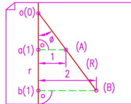
Abatimiento de la recta
