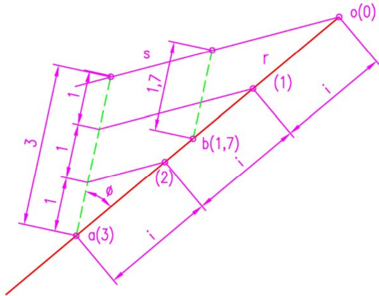
Graduación de la recta
