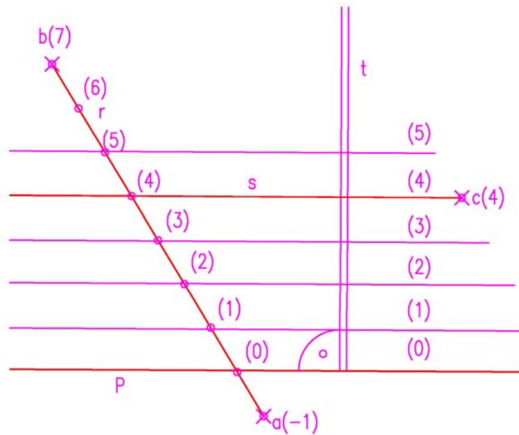
Determinación de un plano
