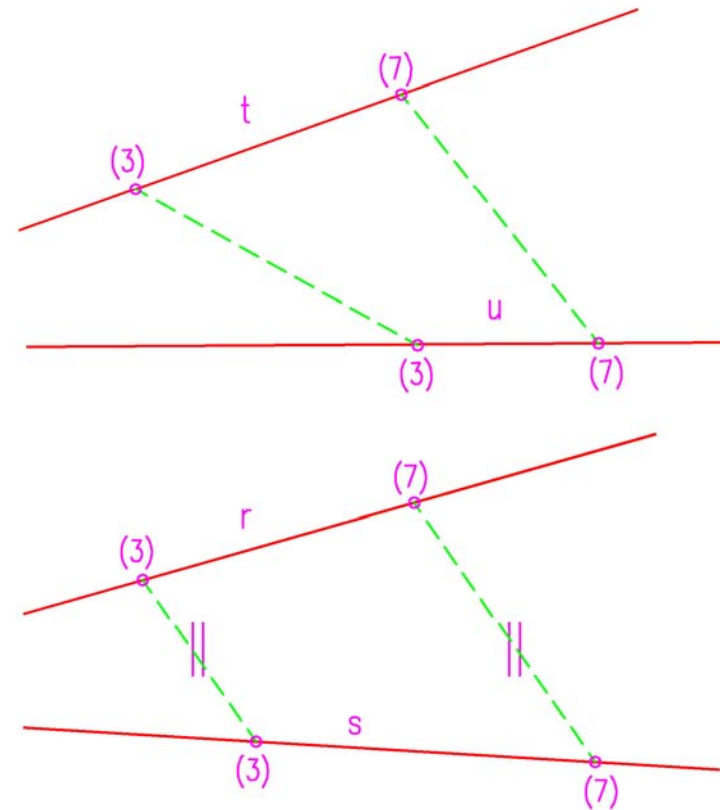
Corte y cruce de rectas
