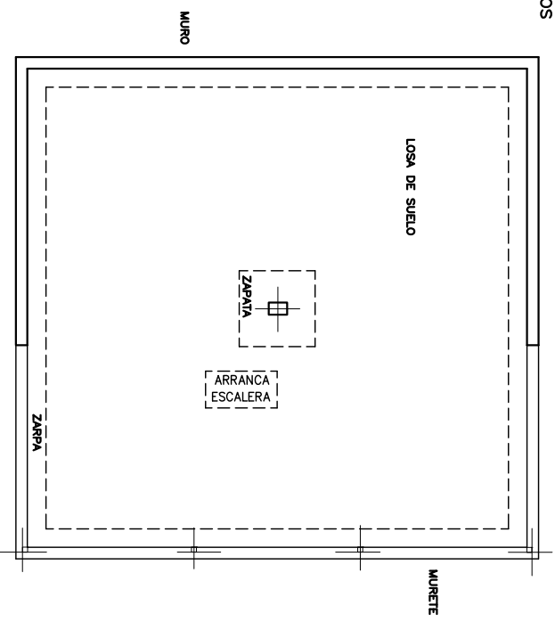
PLANTA DE CIMIENTOS
