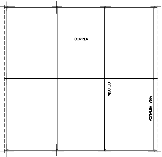
PLANTA DE CUBIERTA
